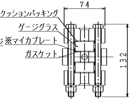
SECTION A-A ※ボイラー用に付属
