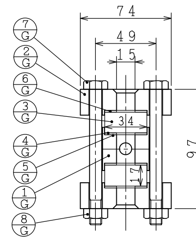
断面 A-A'
