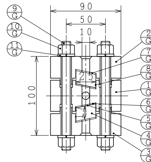
断面 A-A'
